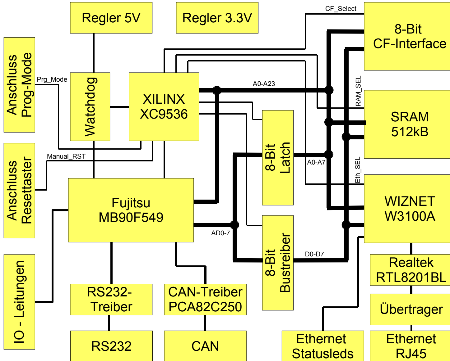
Blockschaltbild: TW-MB549-WZ1-0
